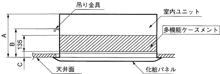
変化寸法表
