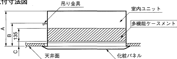
変化寸法表
