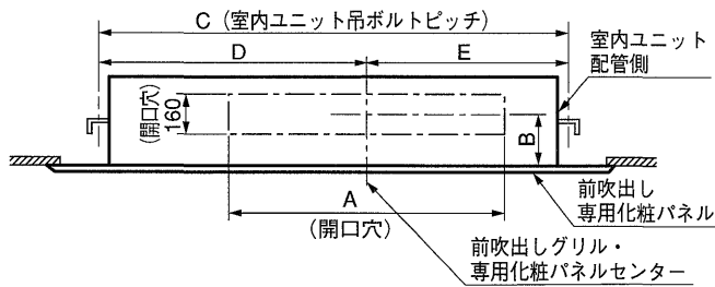
変化寸法表
