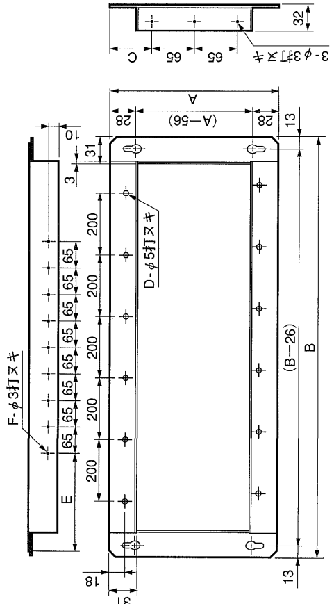
角ダクトフランジ
