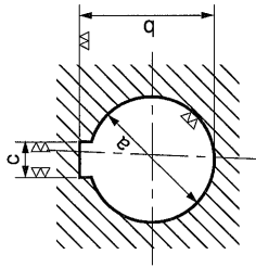
ボス部形状
