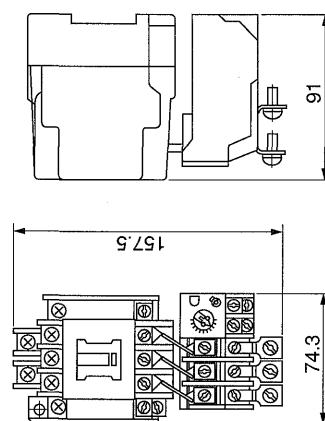
電磁開閉器 MSO-N25, 35 : 三菱電機製 (PAC-CV59~71MPに付属)
