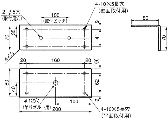
取付用金具
