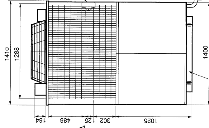
正面図
