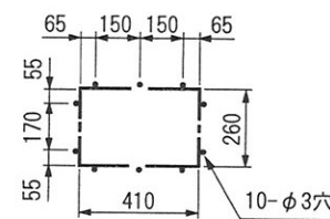
分ダクト穴詳細
