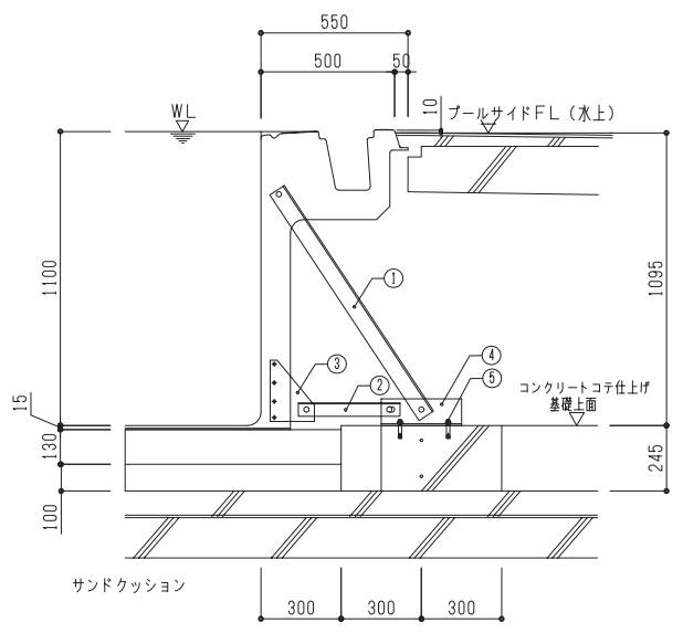
ステー取付詳細図 1/20
