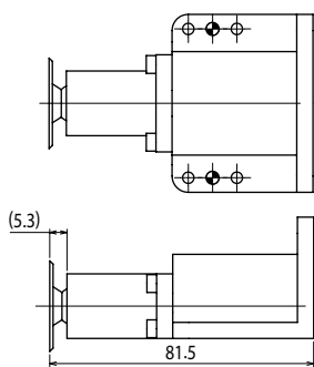
マーク寸法
