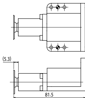
マーク寸法
