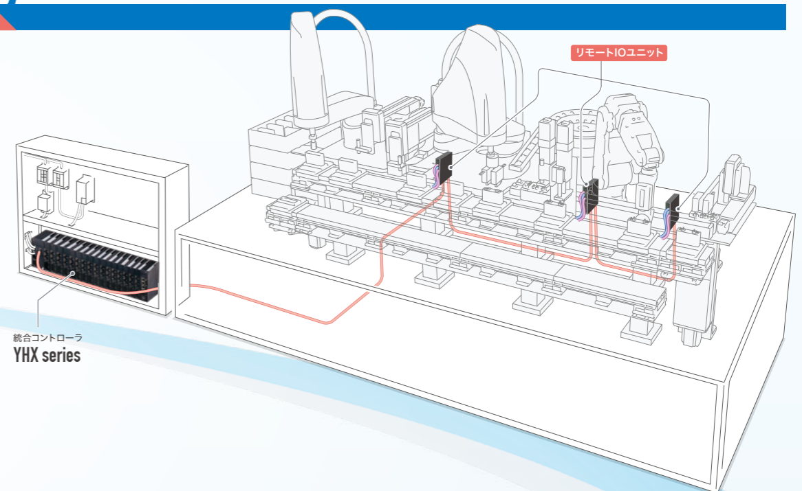
YHXシステム リモートIOユニットの配線
