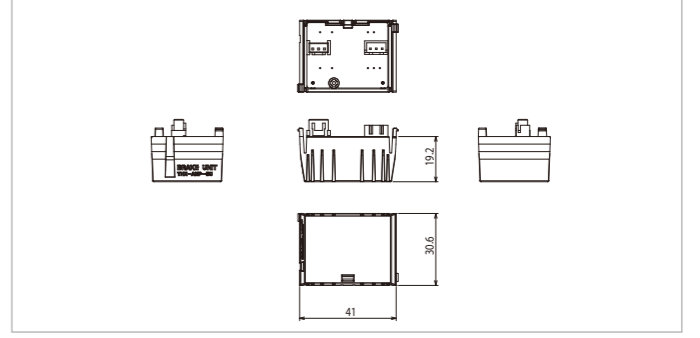
ブレーキユニット YHX-AMP-BU KEK-M5317-00
