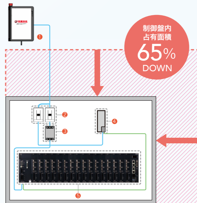
下記の16軸構成の場合の盤内配線の比較 (ロボットケーブルは除く)
