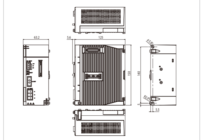
ドライバパワーユニット YHX-DPU KEK-M5880-0A
