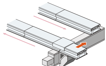
乗り継ぎの途中で循環部を移動
