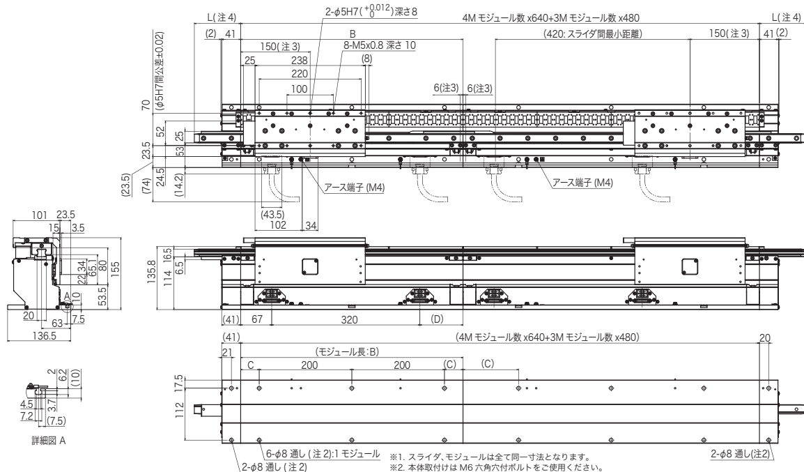
挿入排出レール長選択表
