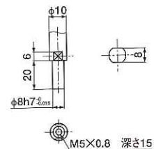
先端部詳細図
